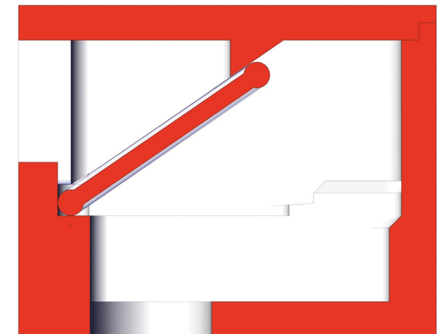
Klappen geschlossen (bei zu hohem Winddruck)
