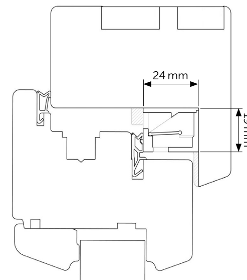
Querschnitt eines Holzfensters mit und ohne arimeo
