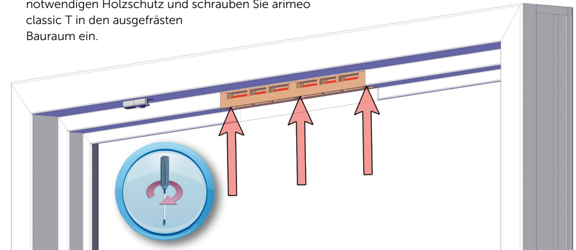
Abbildung 2: Einschrauben von arimeo CT
