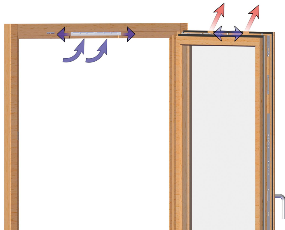
Funktionsprinzip/ Luftführung
