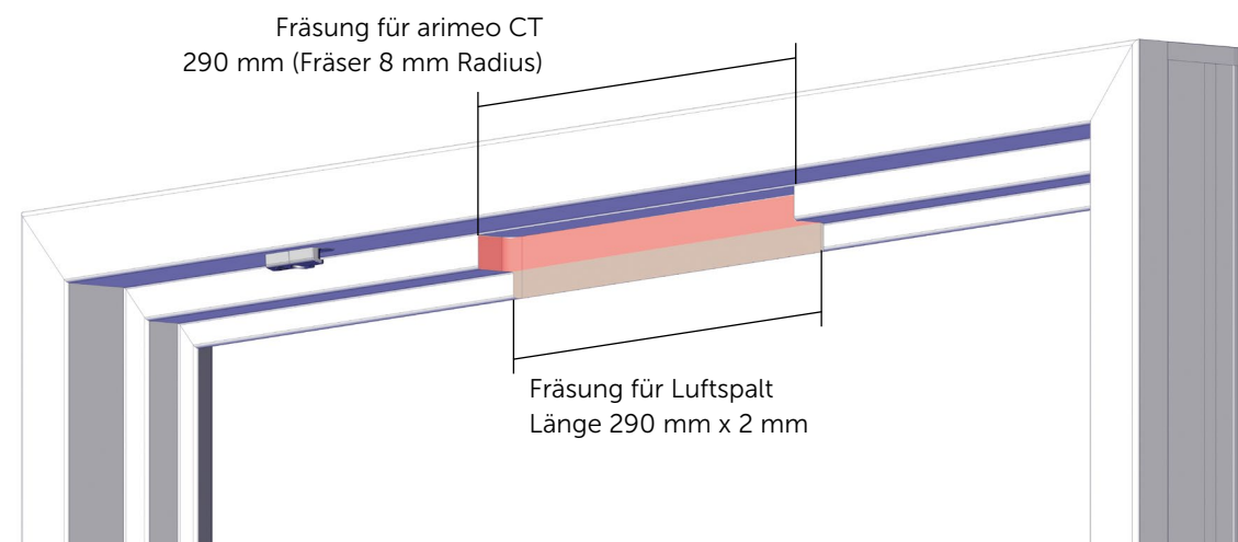
Abbildung 1: Fräsung
